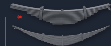
■ Многолистовые (классические) рессоры и листы к ним
